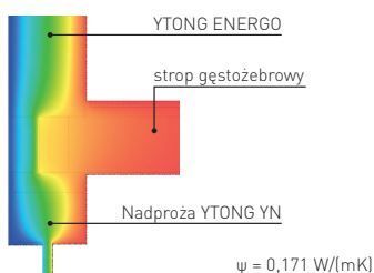
Nadproże YTONG – brak mostków termicznych
